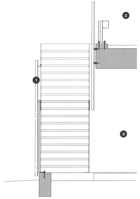
Querschnitt Treppe mit Ansicht an T-Profile.
