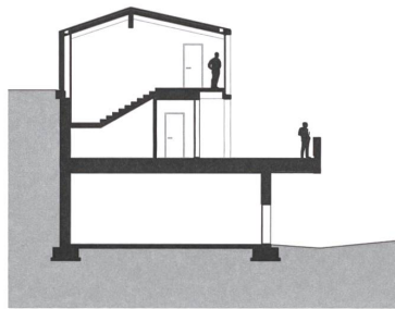
Querschnitt | Section
