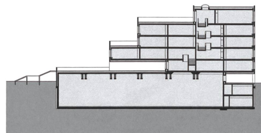
Längsschnitt
