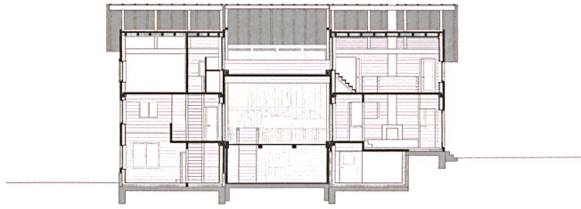
Längsschnitt
