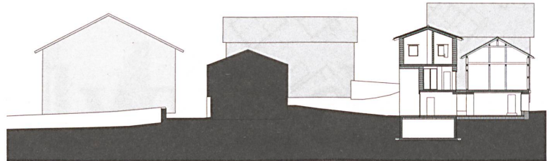
Querschnitt
