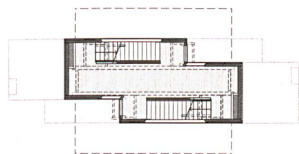
5. Obergeschoss
