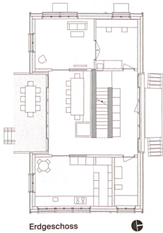
Erdgeschoss
