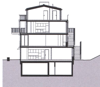
Querschnitt 0 5 10 m
