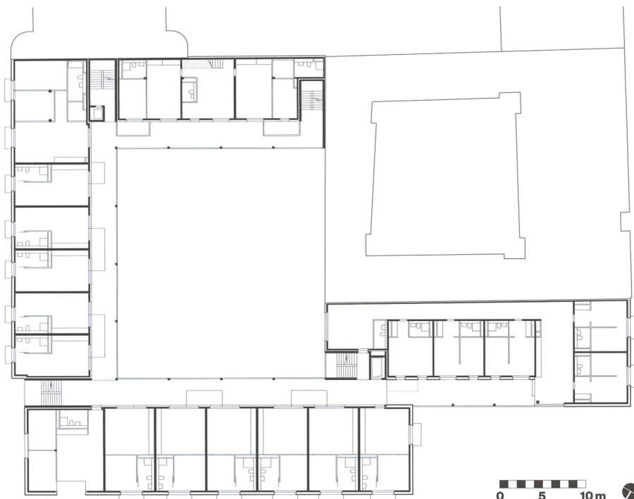
1.-3. Obergeschoss
