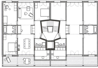
Wohnungstyp Obergeschoss S-Haus.
