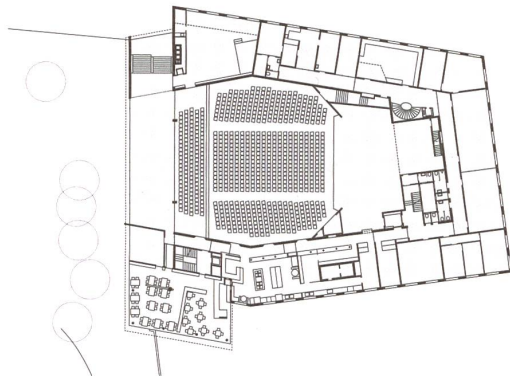
1. Obergeschoss
