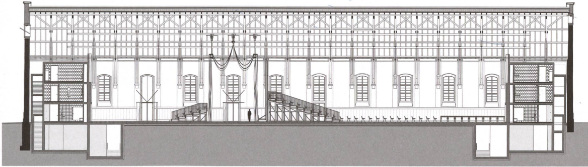
Längsschnitt
