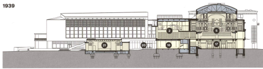
Langschnitt
