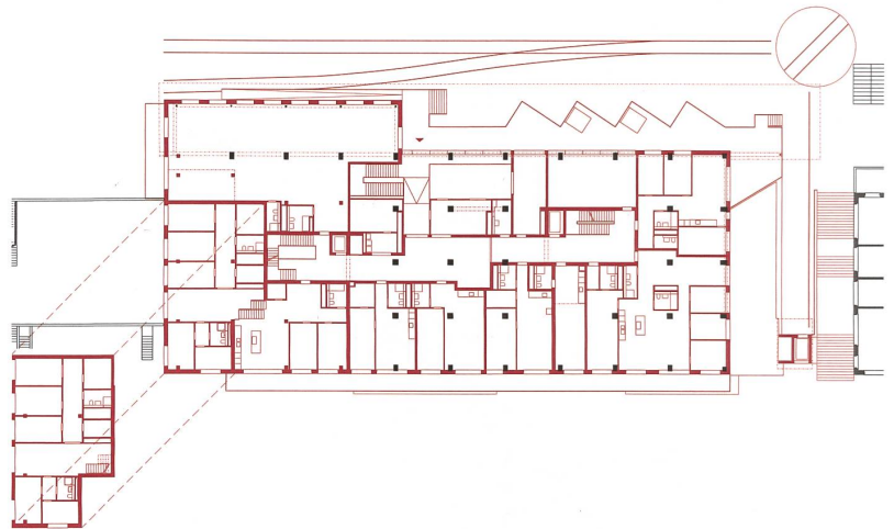
Erdgeschoss
