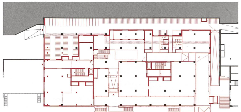
Oberes Hofgeschoss
