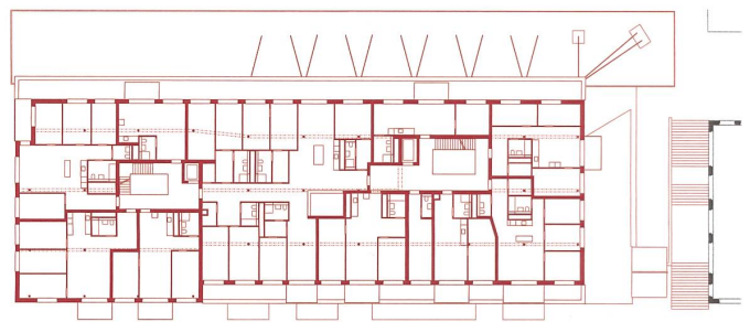
4./5. Obergeschoss
