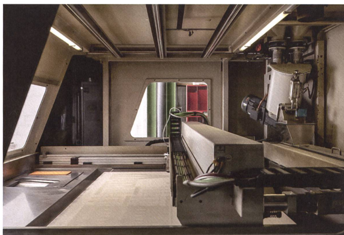
Der 3-D-Drucker kann in kurzer Zeit komplexe Gussformen herstellen.
