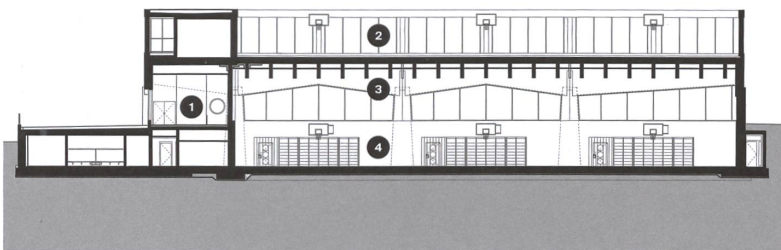
Längsschnitt: Foyer 1, Dachplatz 2, Luftraum 3, Hallen 4.
