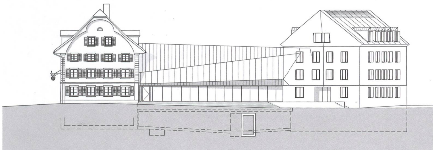
Ansicht Ochsensaal-Wolf
