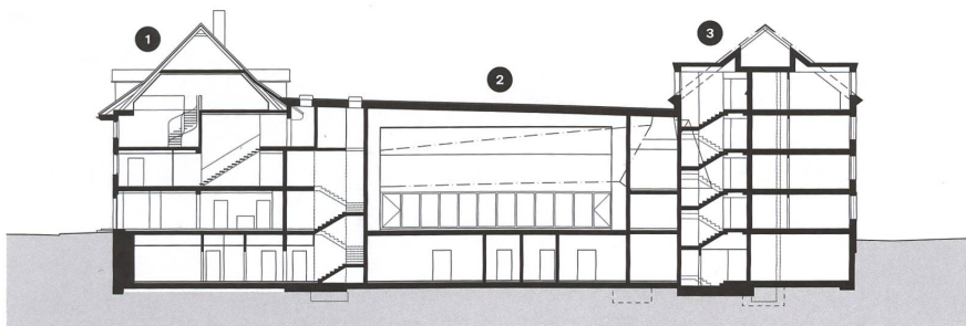
Längsschnitt Ochsensaal-Wolf
