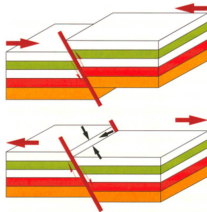
Faulle inverse (en haut), faille normale (en bas).
