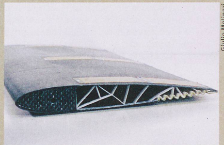
L'aile déformable de l'ETH Zurich agit comme un aileron avec une résistance de l'air réduite.
