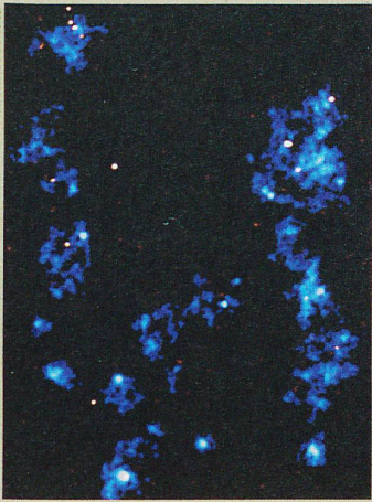
Deux gigantesques filaments de gaz (bleus) alimentent des galaxies (points blancs).
