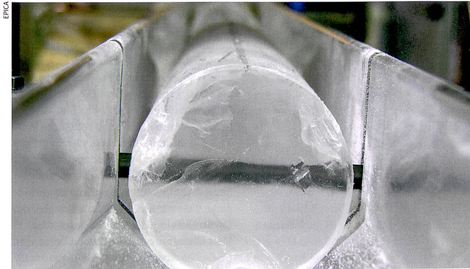
Sensibler Kreislauf: Seine Veränderungen lassen sich an Eisbohrkernen ablesen.
