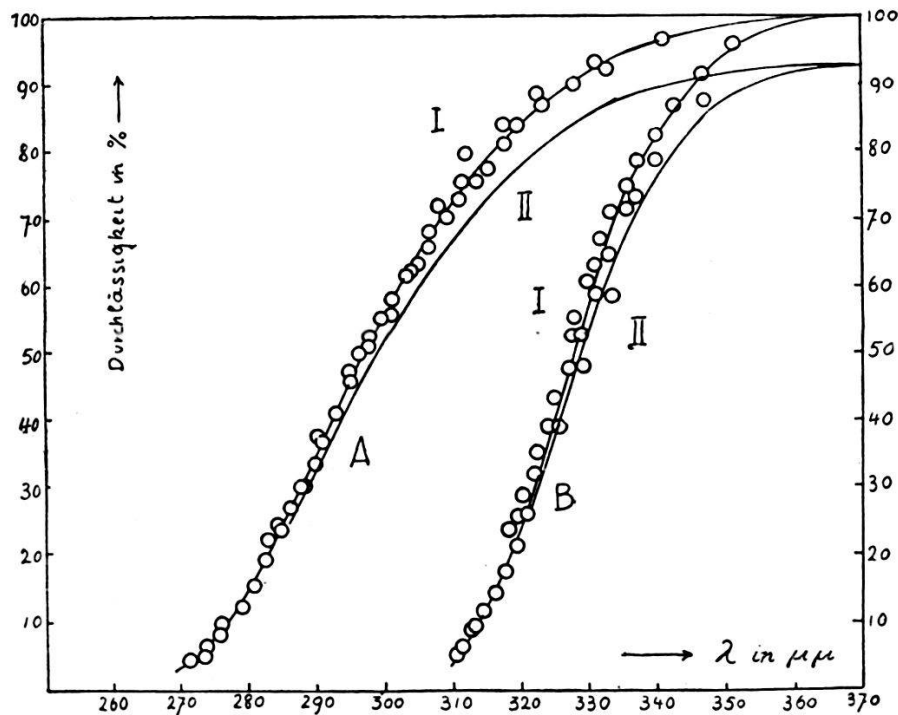
Fig. 10. Durchlässigkeitskurven für „Ultravitlease“ und belg. Fensterglas (I ohne Reflexionsverluste; II. mit Reflexionsverlusten).
