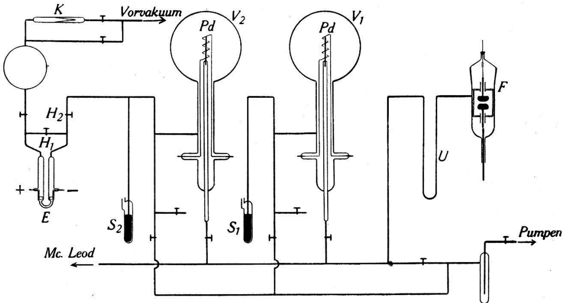
Fig. 2. Glasapparatur.
