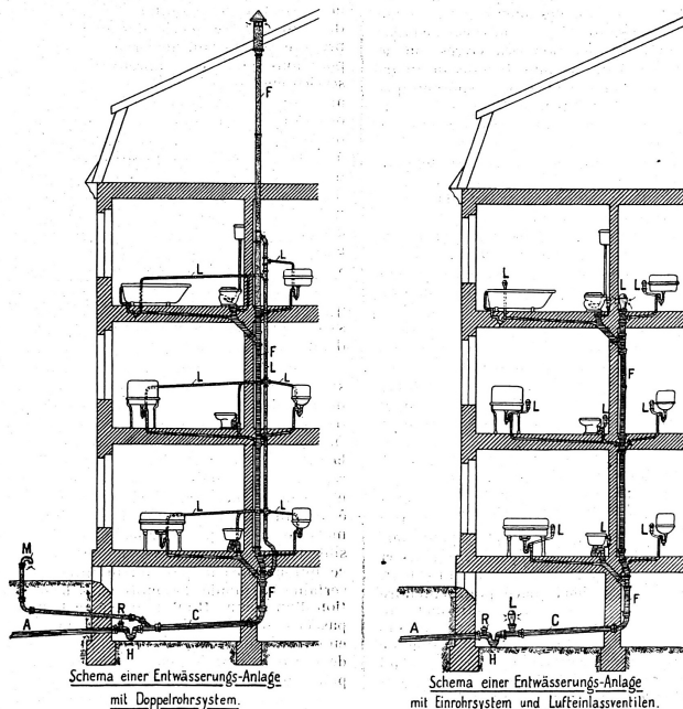
Fig. 4. Schema einer Entwässerungs-Anlage mit Doppelrohrsystem. A. Anschlussrohr an den Strassenkanal. C. Hauskanal. F. Abfallrohr. N. Hauptwasserschluss. L. Lüftungsrohr. M. Mündung des Frischluftrohres. R. Reinigungsöffnung. Fig. 5. Schema einer Entwässerungs-Anlage mit Einrohrsystem und Luftleinlassventilen. A. Anschlussrohr an den Strassenkanal. C. Hauskanal. F. Abfallrohr. H. Hauptwasserschluss. L. Luftleinlassventile. R. Reinigungsöffnung.
