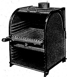
Elektrischer Grill-Salamander in der Stellung zum Grillieren
