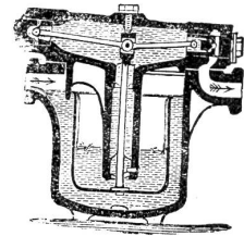
Condensationstöpfe
