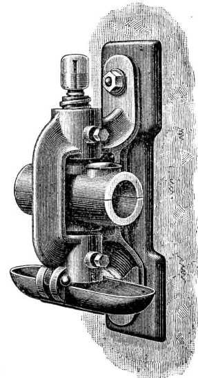
Geschlossenes Wandlager
