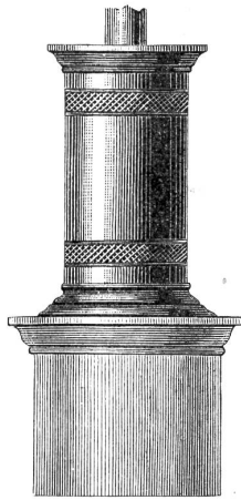
Ofensäule mit Doppel- mantel, Luftzirkulation und drei Ranchzügen.
