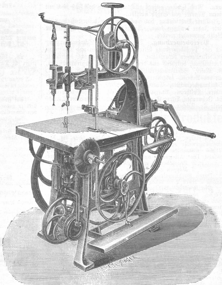
Universal-Holzbearbeitungs-Maschine.
