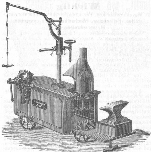
Montirapparat , ganz Eisenkonstruktion, drehbarem Hebel zum Ziehen und Treten. Mit zwei geräumigen, verstellbaren Werkzeugkästen, Kohlenkasten, Schraubstock, Bohrmaschine, Ambos sammt Vorrichtung dazu.
