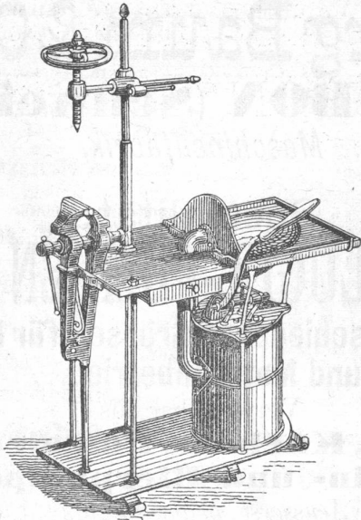
Feldschmiede mit Werkbisch, Schublade, Schraubstock und Bohrmaschine, mit drehbarem Hebel zum Drücken oder zum Ziehen; Tisch und Bodenplatte aus Schmiedeeisen, Gasse und Deckplatte aus Gußeisen.
