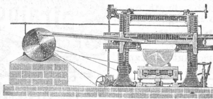
Horizontal-Sägegatter.
