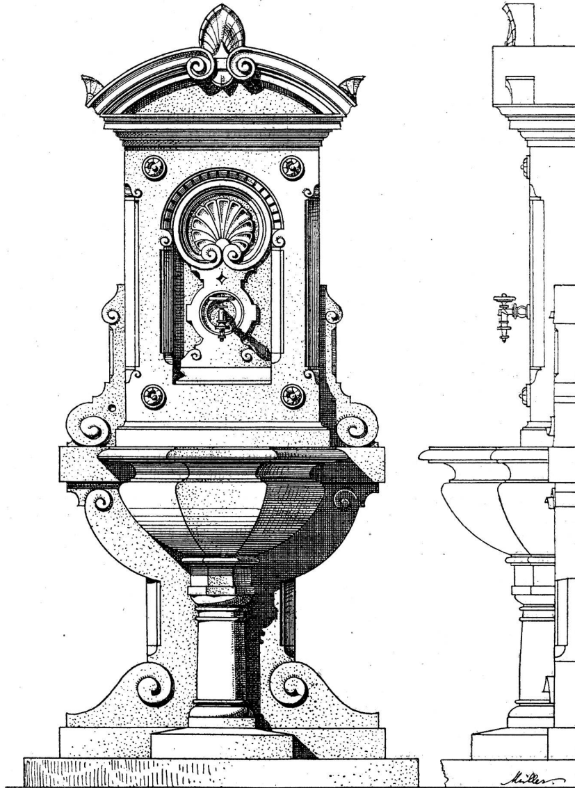
Wandbrunnen aus Stein. ( \frac{1}{5} natürlicher Größe.) Entworfen von Gewerbelehrer H. Müller.
