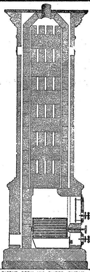
PATENT-OFEN MIT SUTER-EINBAU. SUTER-OFEN. POÛLE SUTER, BREVETÉ (S. D. O. G.) COUPE TRANSVERSALE.
