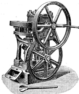
Excenterpresse
