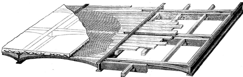
Fig. 11. Goldings Deckenkonstruktion.
