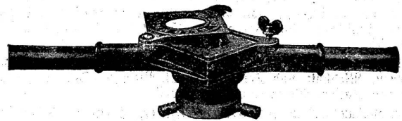
Fig. 4. Reed's Rohrschneidkluppe.
