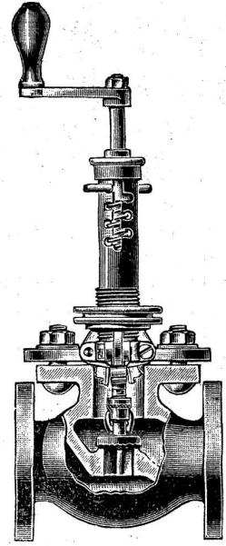
Fig. 4. Ausschleifen des Ventiltiegels auf den Ventilsitz.
