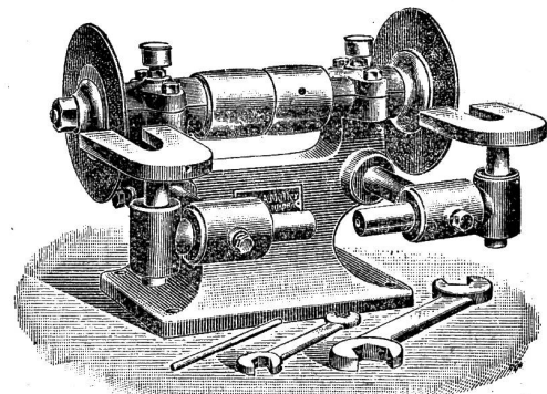
Kehlmesserschleifapparat
