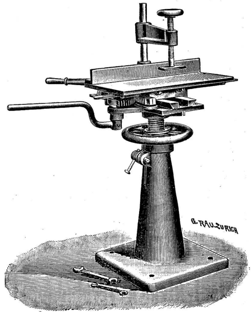
Bohrständer
