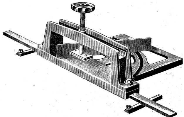
Zapfenschneidtischen
