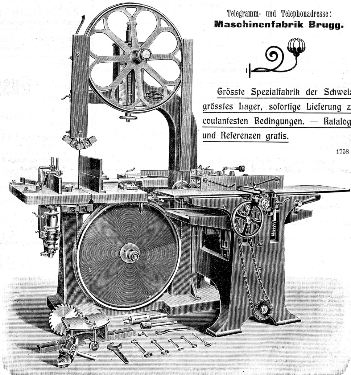
Universalsmaschine No. 3.
