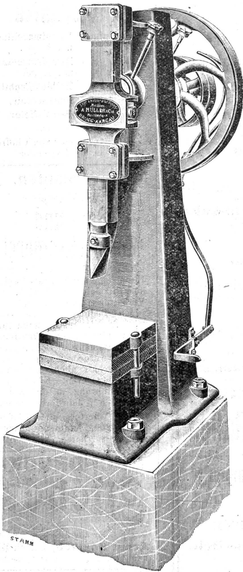
Holz-Spaltmaschine
