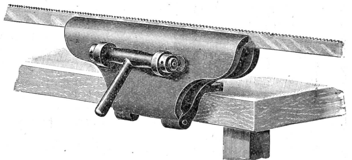
Feilschraubstock
