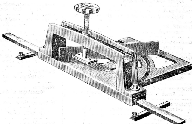
Zapfenschneidmaschine
