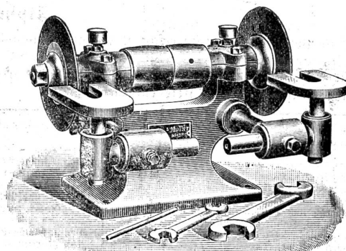
Kehlmesserschleifapparat
