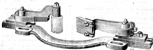
Kehlandruckapparat
