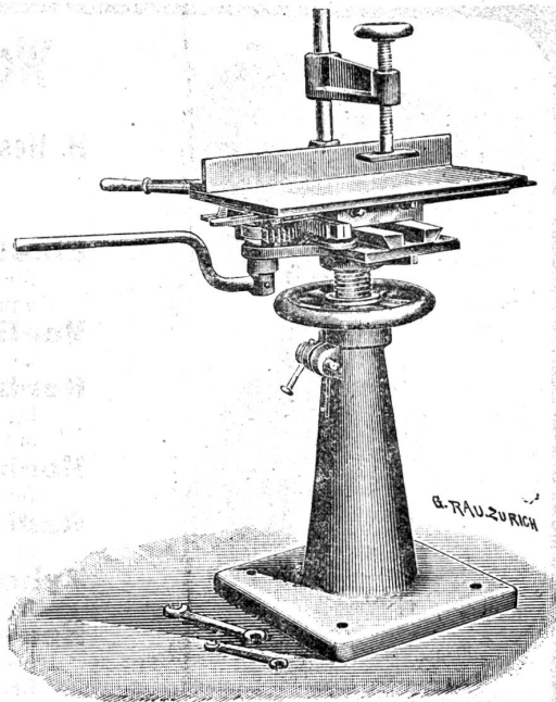
Bohrständer
