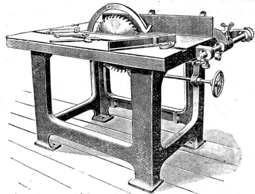
Kreissäge
