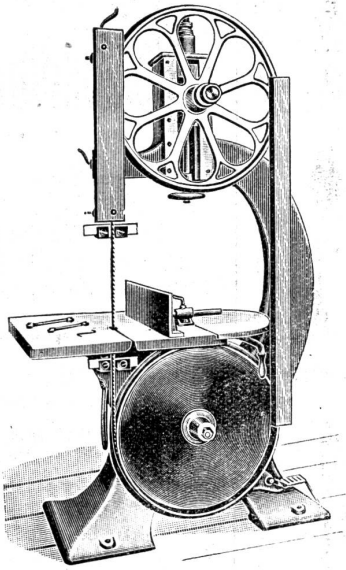
Kleinere Bandsäge.
