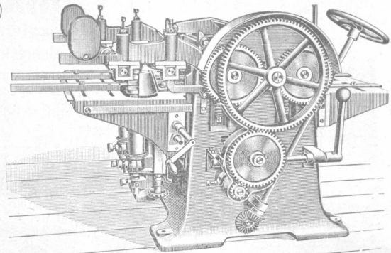
Dreiseitige Hobelmaschine.
