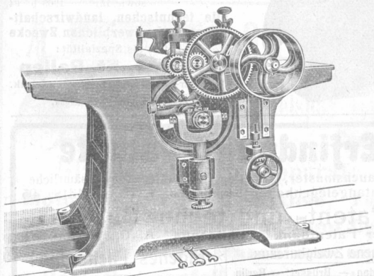
Sandpapierschleifmaschine
