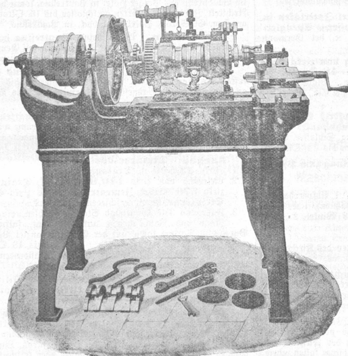
Fräser-Hinter-Drehbank.
