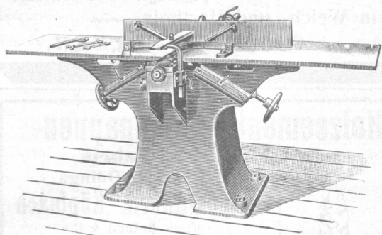
Abrichtmaschine.
