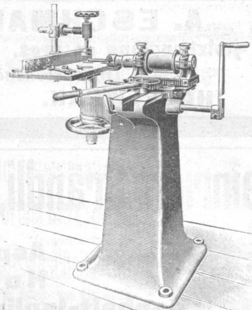
Langlochbohrmaschine.
