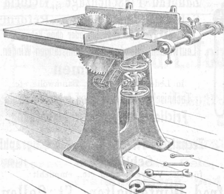
Kreissäge
