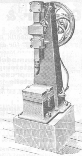
Holzspaltmaschine.
