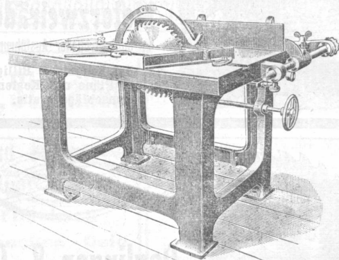
Kreissäge
