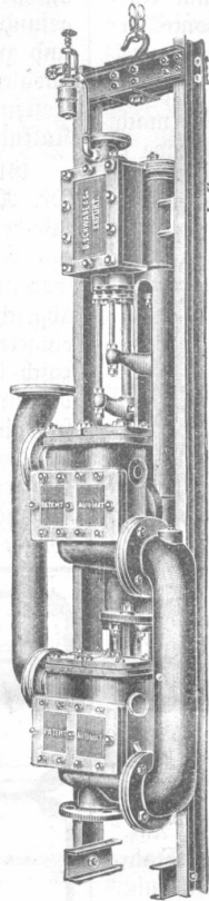
Fig. 5. Abteufelpumpe.
