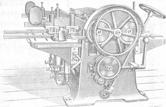
Dreiseitige Hobelmaschine.
