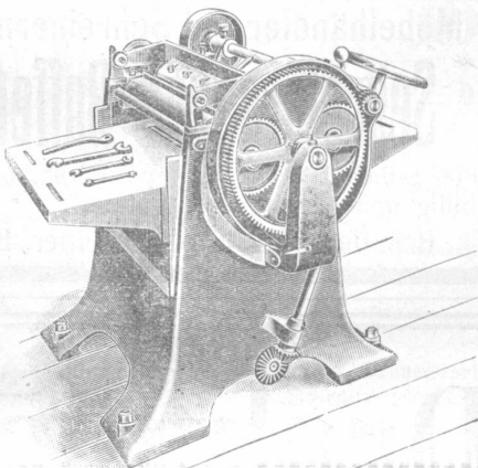
Dickehobelmaschine.
