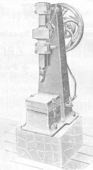
Holzsplattmaschine.
