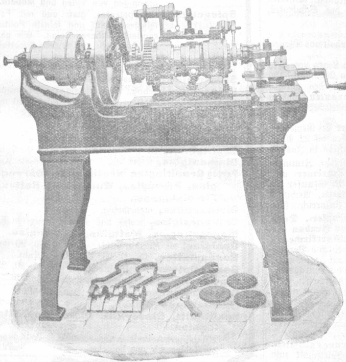
Fräser-Hinter-Drehbank.
