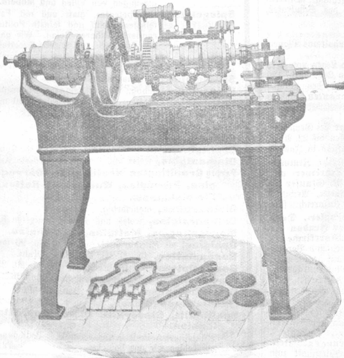
Fräser-Hinter-Drehbank.
